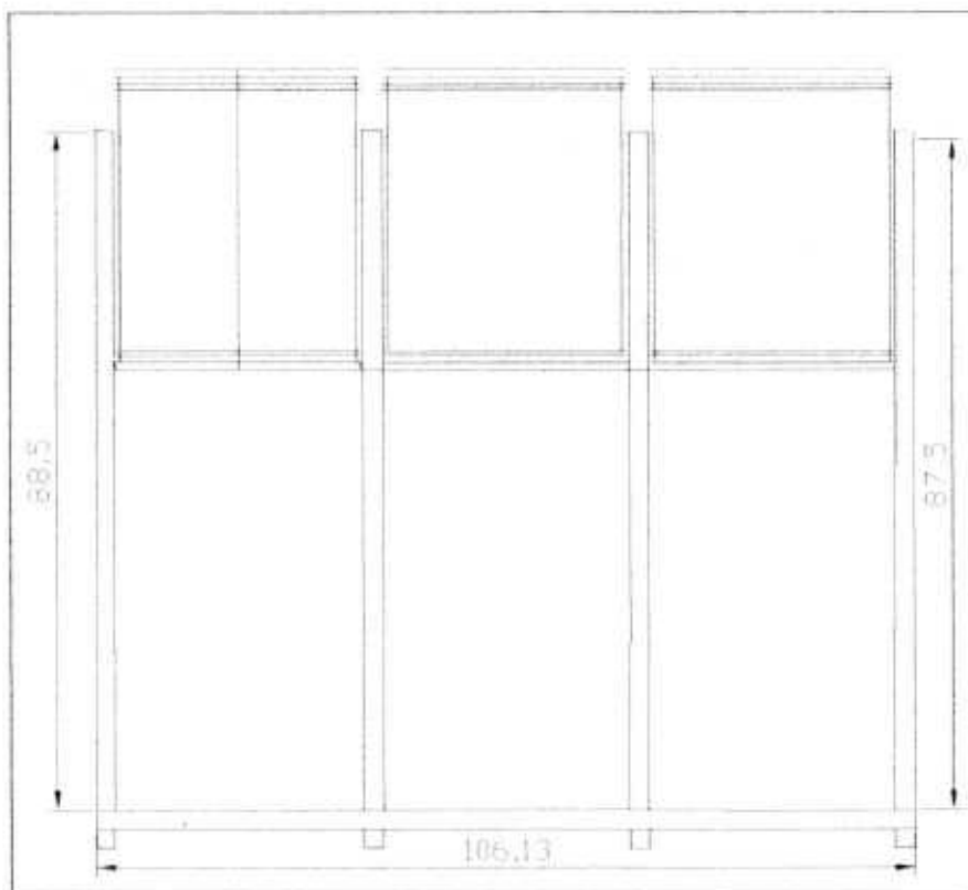
VISTA FRONTAL. E=1:10
